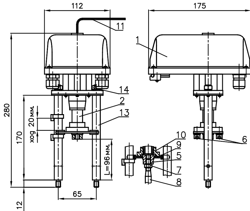
Рисунок 1 - ВЭП-111-1600
