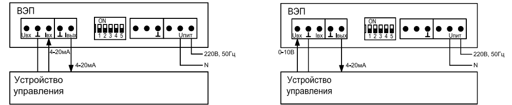
Рисунок 3 - Схема подключения ВЭП-138М в режиме управления аналоговым сигналом 4-20 мА (0-10 В)
