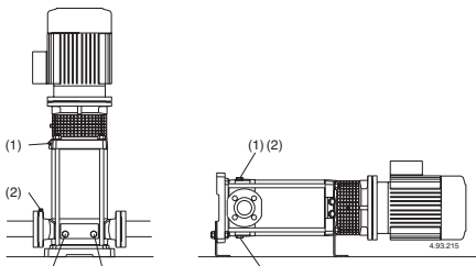
ΕΣΧ. 4 (1) Γέμισμα και εξαέρωση (2) πρόσληψη εξαερισμού (3) Αποστράγγιση
