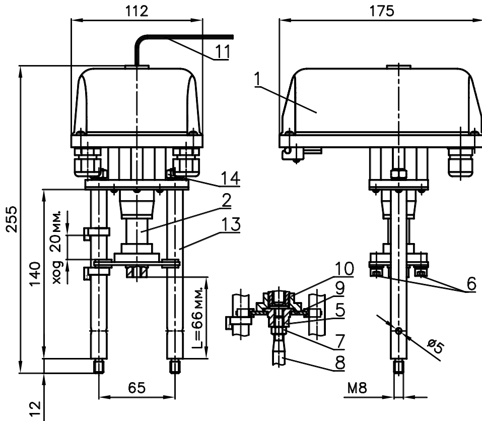
Рисунок 1 - ВЭП-115М-1600
