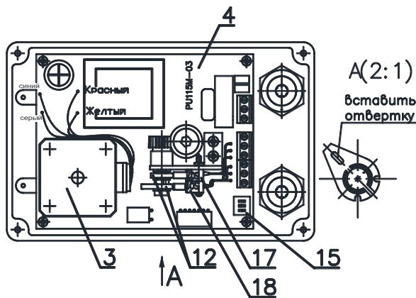
Рисунок 2 - Электропривод (вид при снятой крышке)
