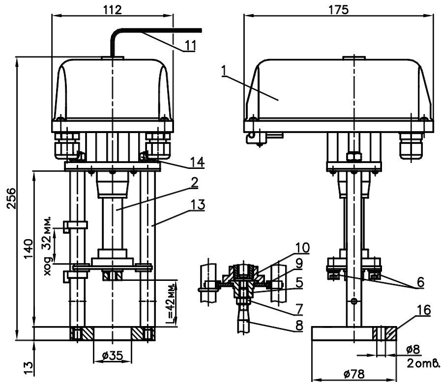
Рисунок 1 - ВЭП-118М-2700
