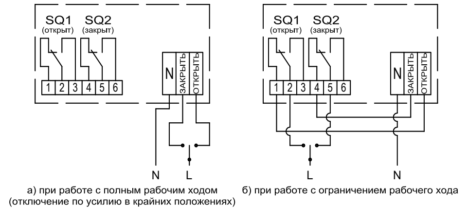
Рисунок 3 - Схема подключения
