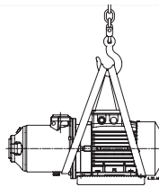
Fig. 7 Sollevamento pompa Raising the pump Anhebung Pumpe Suoilevament de la pompe Elevación de la bomba 吊起水泵
